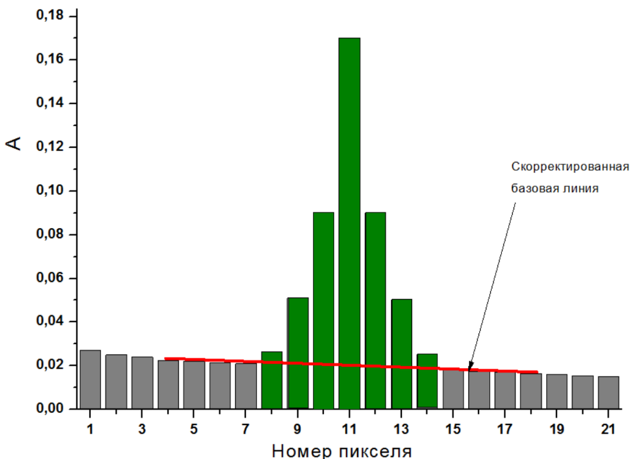
Рис 44. Вид спектра при использовании в качестве приемника излучения линейки ПЗС. Пиксели 8-14 (выделены зеленым) формируют контур спектральной линии. Пиксели 4-7 и 15-18 используются для коррекции базовой линии.
