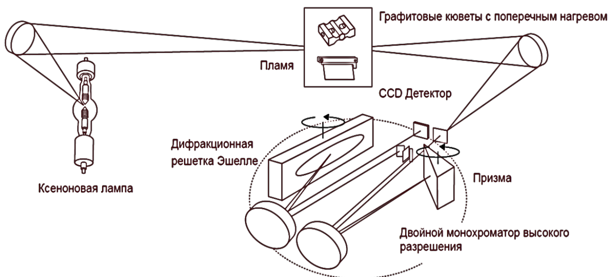
Рис 42. Схема спектрометра ContrAA.
