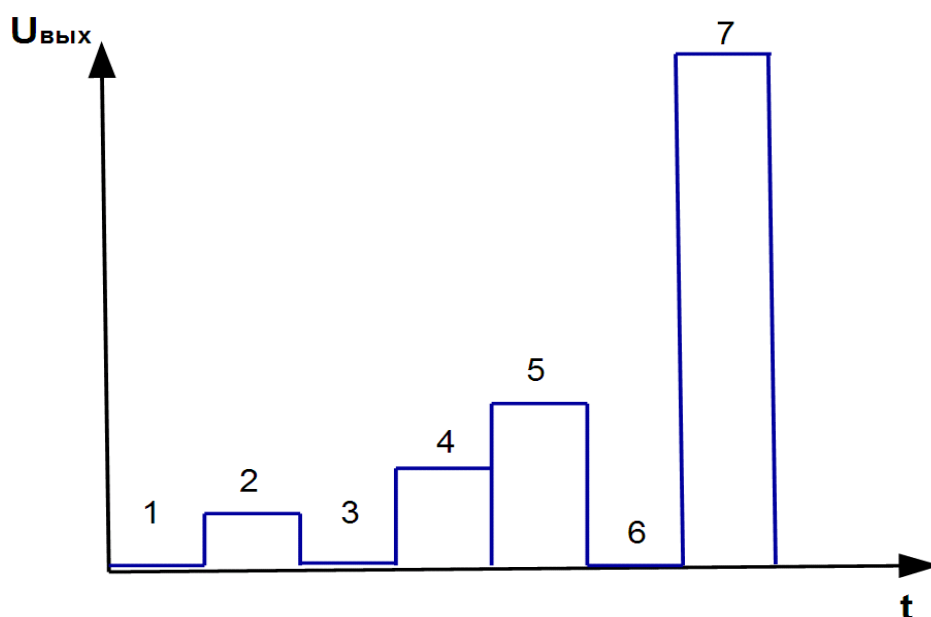
Рис. 23. Формирование пакета выходных данных считывающего устройства ПЗС. Нумерация импульсов соответствует номерам пикселей на рис.22.
