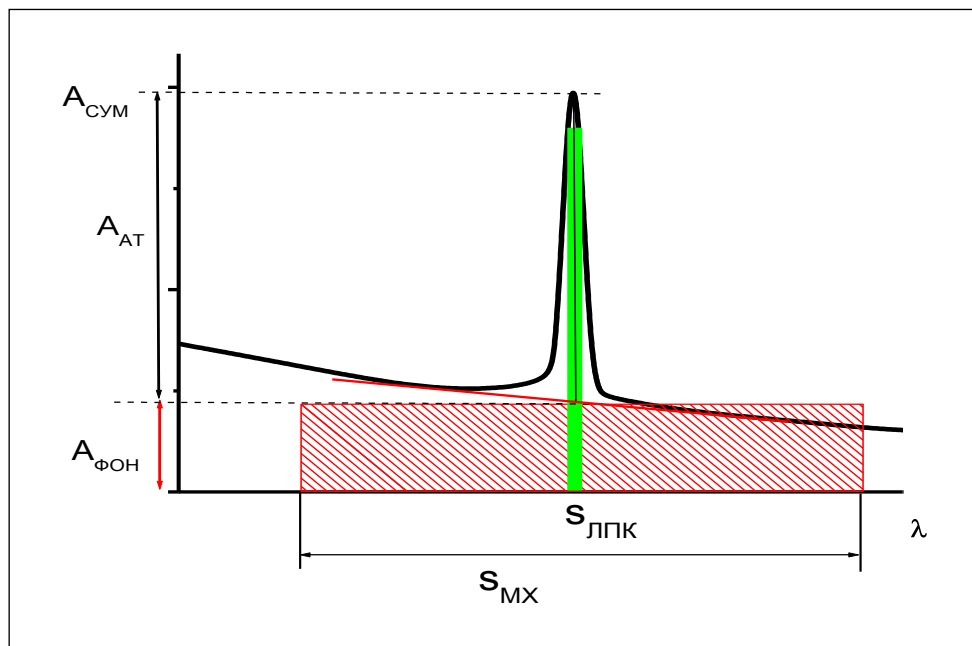
Рис. 38. К методам компенсации неселективного поглощения с использованием дейтериевого корректора. s_{МХ} - интервал \lambda , пропускаемый монохроматором, s_{ЛПК} - ширина линии ЛПК. Измерение при s_{ЛПК} дает суммарную оптическую плотность A_{СУМ} , при s_{МХ} - близкую к оптической плотности фона A_{ФОН}
