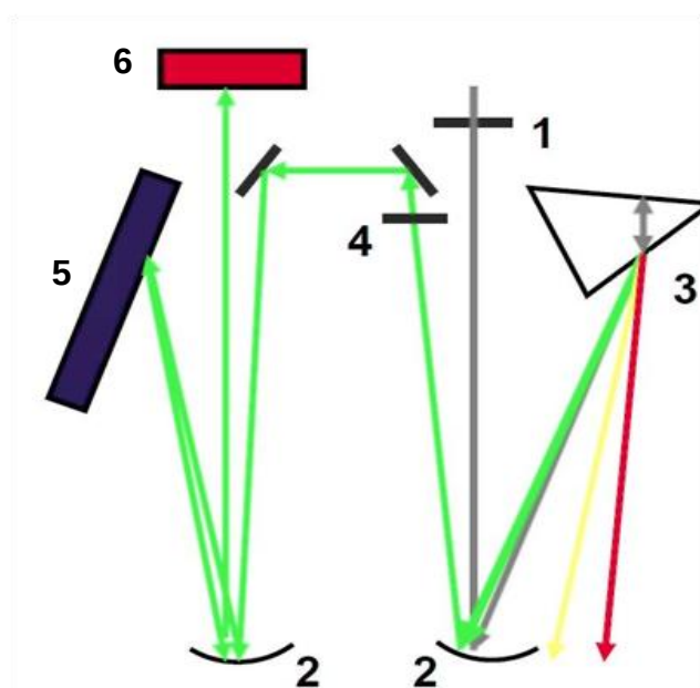
Рис 43. Схема монохроматора contrAA. 1 – входная щель, 2 – зеркала, 3 – призма Литтрова, 4 – вторая входная щель, 5 – дифракционная решетка, 6 – фотодиодная матрица
