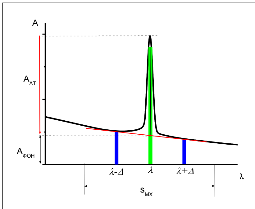
Рис. 40. К методу компенсации неселективного поглощения с использованием эффекта Зеемана. При поляризации излучения под прямым углом к полю при (\lambda - \Delta) и (\lambda + \Delta) измеряется A_{\text{ФОН}} , а при параллельной поляризации – A_{\text{СУМ}} (при длине волны \lambda )
