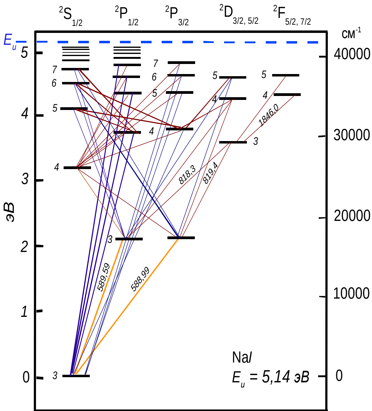
Рис. 4. Схема Гроттриана для атома натрия. E_u – энергия ионизации
