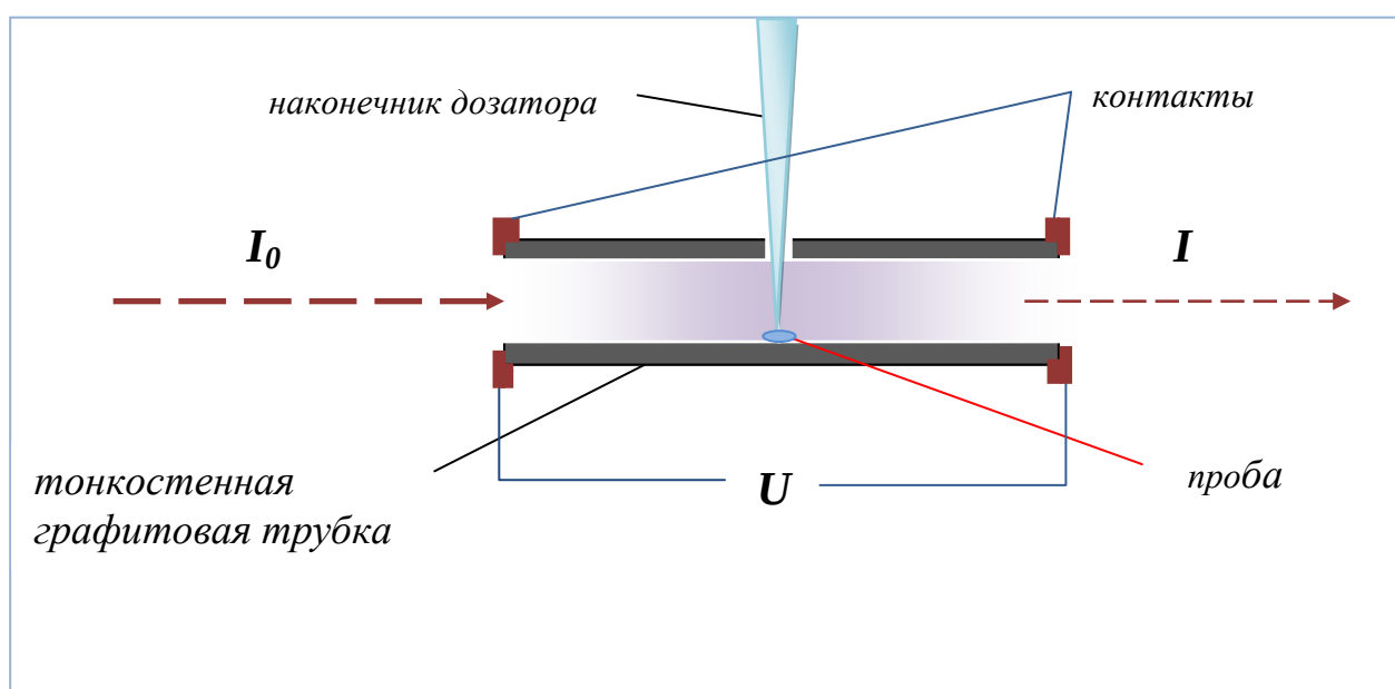
Рис. 34. Графитовая печь Массмана
