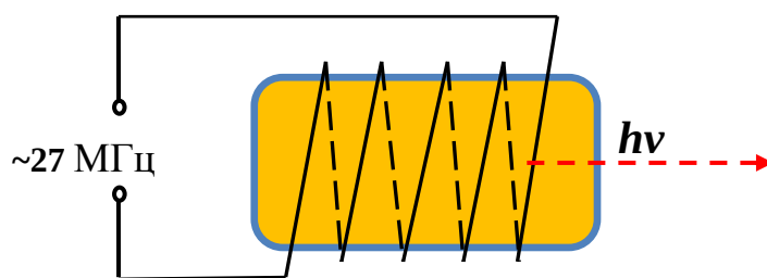
Рис. 30. Устройство высокочастотной газоразрядной лампы
