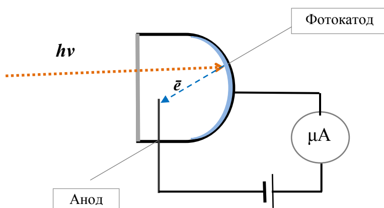
Рис. 20. Вакуумный фотоэлемент
