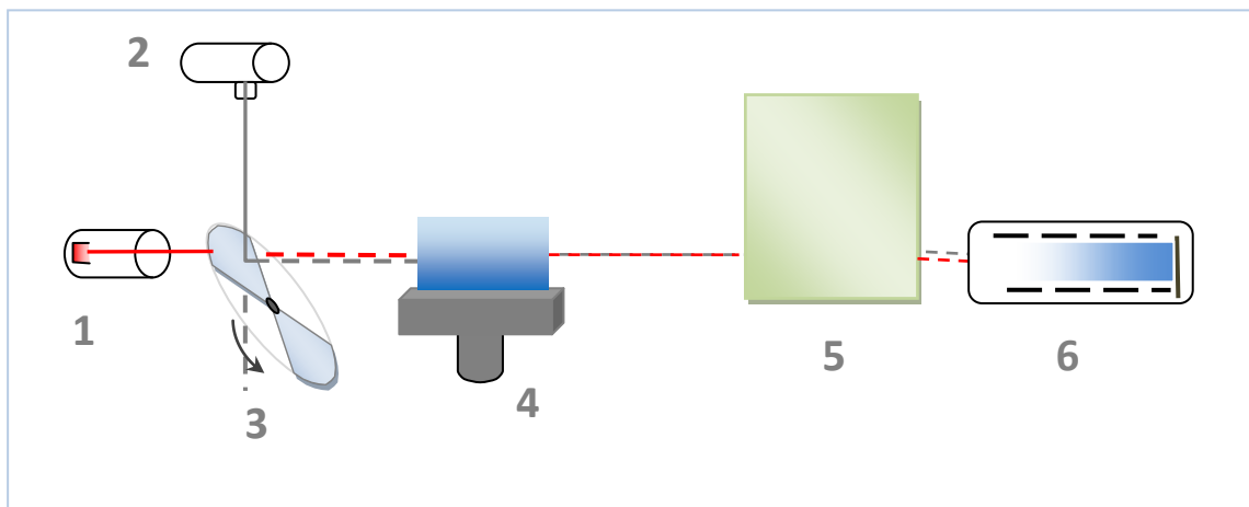
Рис. 39. Схема дейтериевого корректора неселективного поглощения. 1 – ЛСП, 2 – дейтериевая лампа, 3 – прерыватель с зеркальными лопастями, 4 – атомизатор, 5 – монохроматор, 6 – ФЭУ
