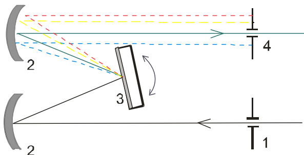
Рис. 17. Монохроматор Черни – Тернера: 1- входная щель, 2 - сферические зеркала, 3 - дифракционная решетка, 4 – выходная щель
