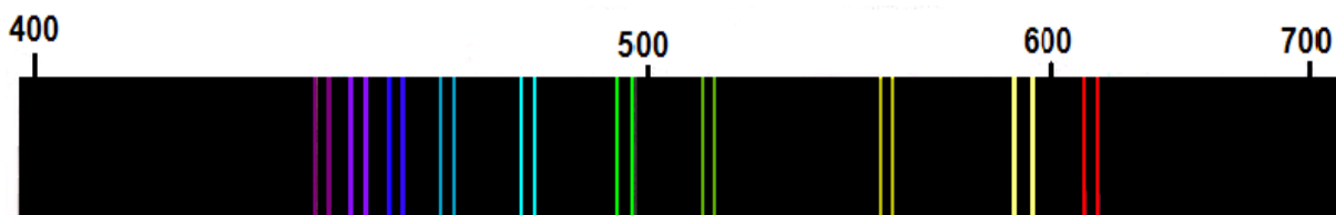
Рис. 2. Эмиссионный спектр паров натрия
